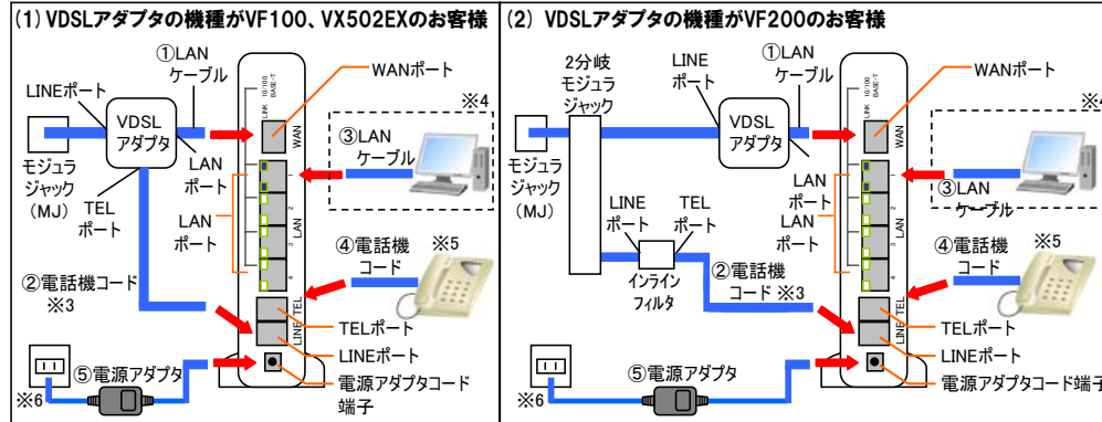
図2：「VDSL方式」
