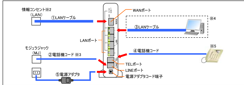
図2：「VDSL方式」
